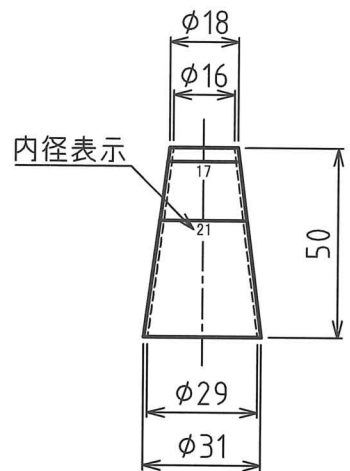
補助ケーブルアーマー HAI-16
