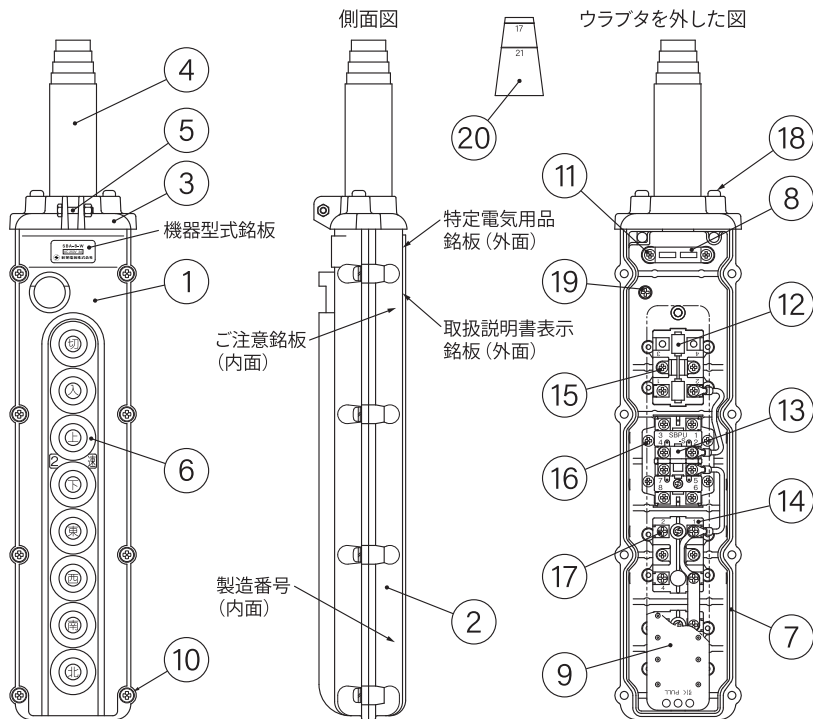
■部品一覧表
