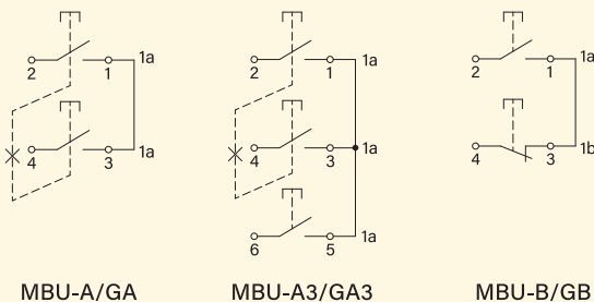
接点構成 (視一端子ねじ側)
