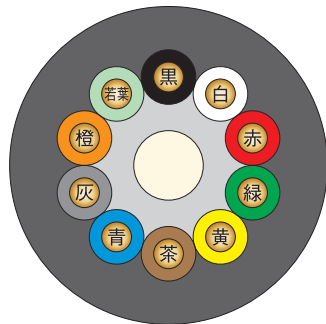
図13-4 10心
