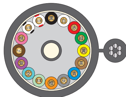
図14-8 16心
