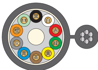
図14-6 10心
