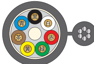
図14-4 7心
