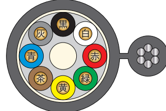
図14-5 8心
