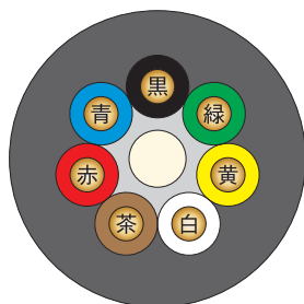
図14-1 複合 SS-VCT
