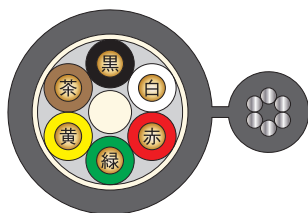
図14-3 6心
