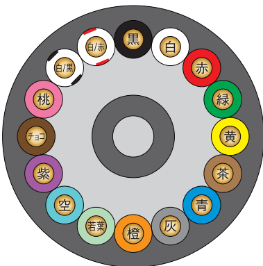
図13-6 16心
