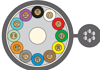
図14-7 12心
