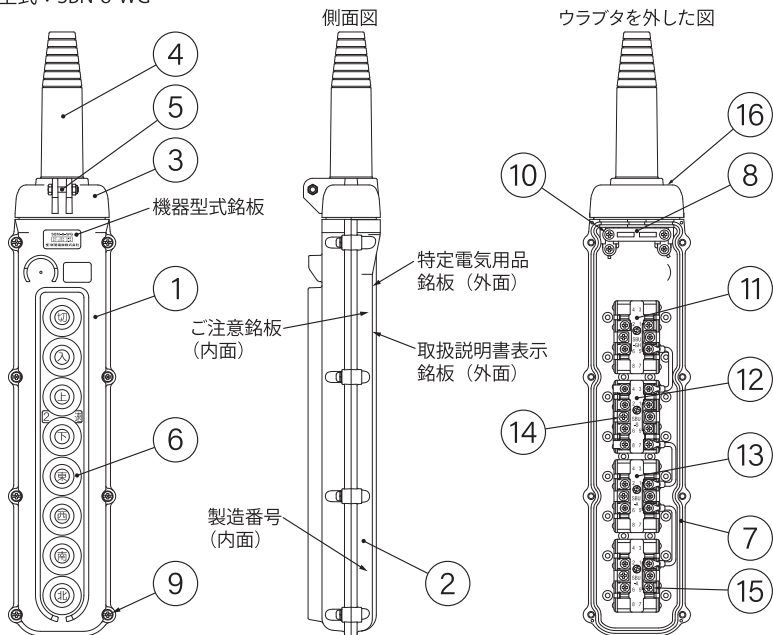
■部品一覧表
