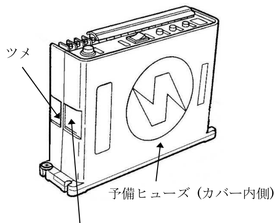
この部分を押さえる (対面側も同じ)
