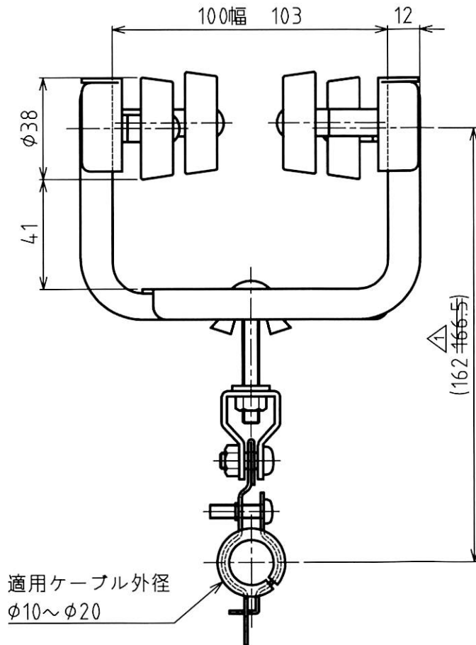
チェーン牽引金具
