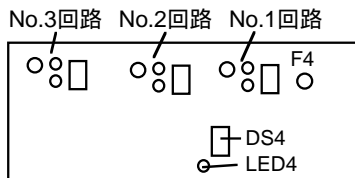
カバーを外した図
